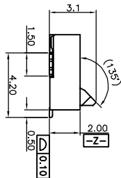
SECTION A-A SCALE 1:1
